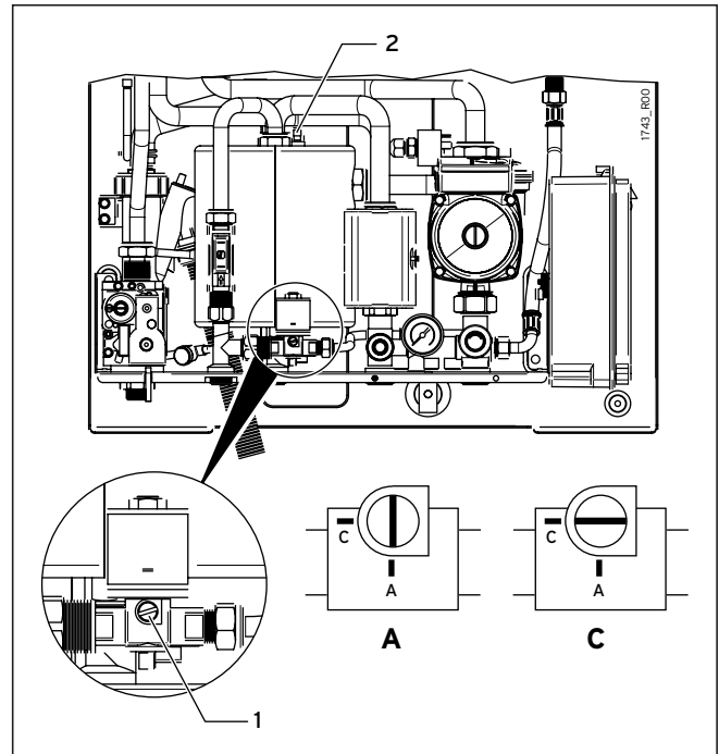
Fig. 5.5 Riempimento impianto
