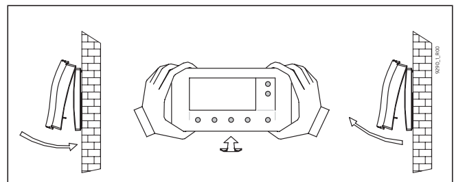
Fig. 5.10 Apertura/chiusura Cronocomando
