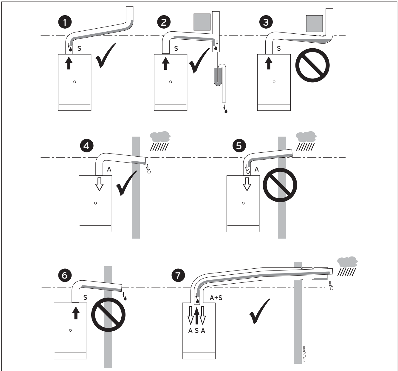
Fig. 5.14 Esempi di installazione condotti di aspirazione/scarico
