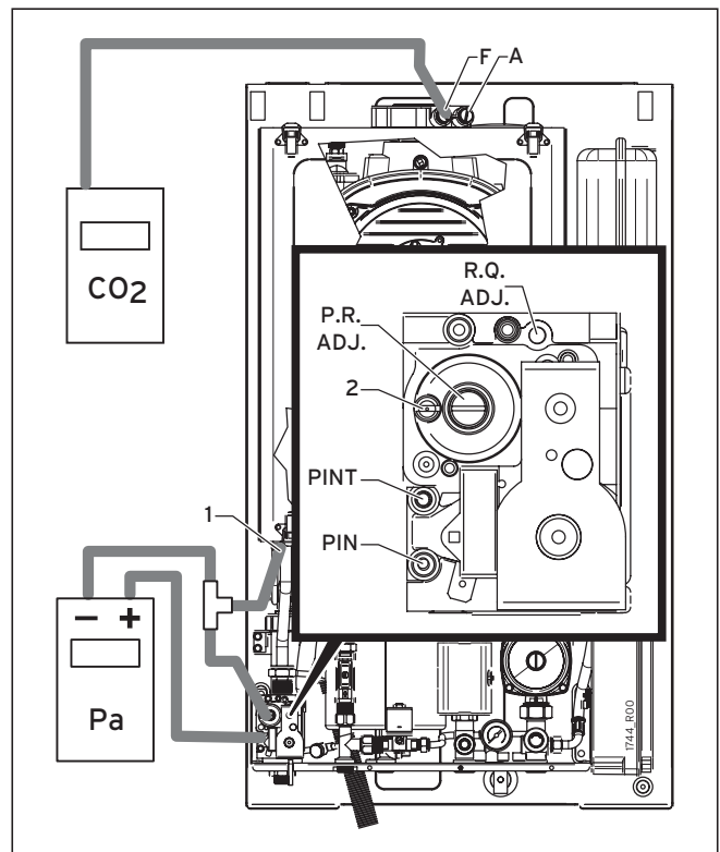
Fig. 6.7 Controllo e regolazione della combustione
