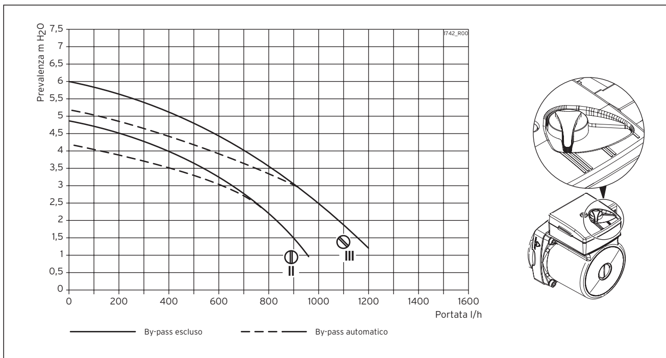
Fig. 10.1 Grafico prevalenza
