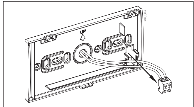
Fig. 5.9 Estrazione e collegamento morsetteria Cronocomando
