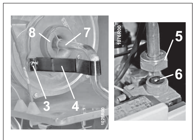
Fig. 6.12 Procedura trasformazione gas
