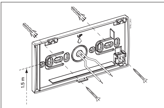
Fig. 5.8 Fissaggio a parete parte posteriore Cronocomando
