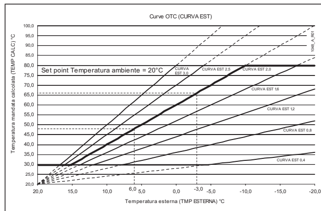
Fig. 6.18 Grafico CURVA EST
