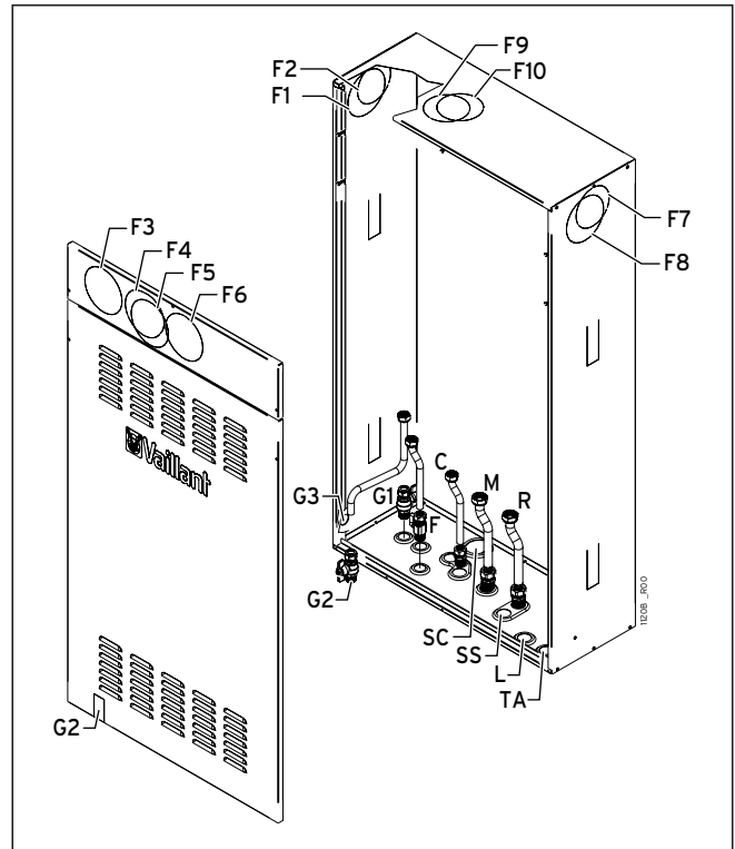
Fig. 5.1 Installazione raccordi
