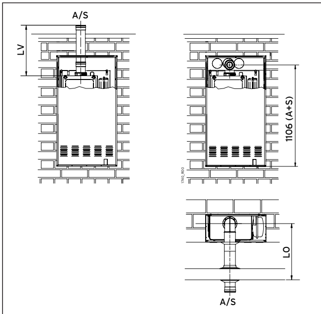
Fig. 5.20 Quote scarichi con sistema coassiale (C 13 e C 33 )
