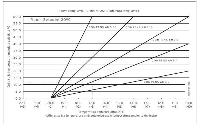
Fig. 6.21 Grafico CURVA Compensazione Ambientale
