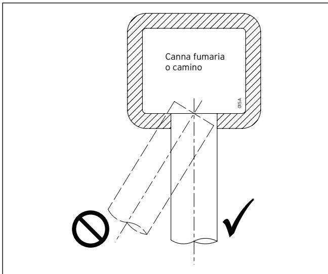
Fig. 5.15 Posizione tubo all'interno della canna fumaria
