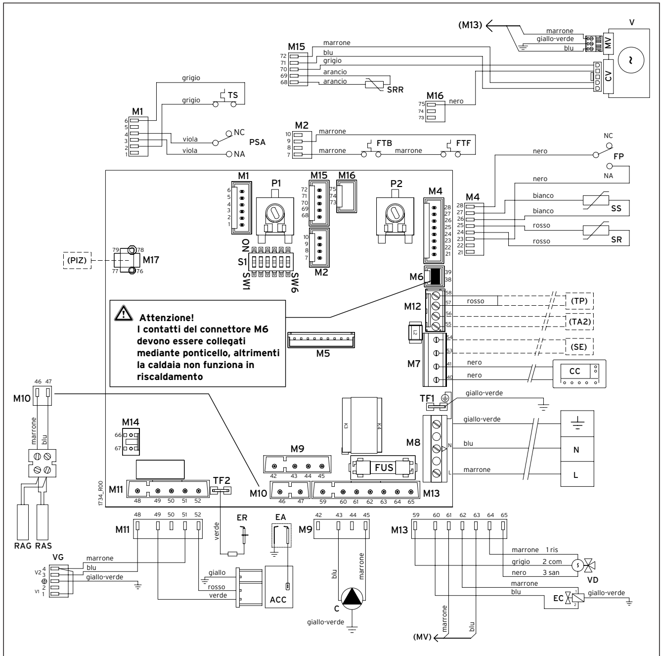
Fig. 5.11 Schema elettrico
