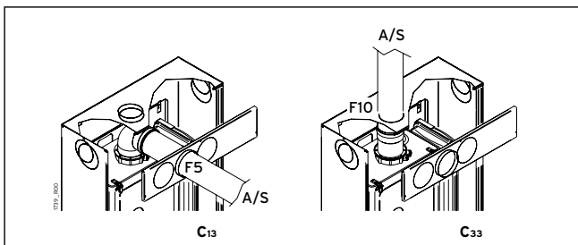
Fig. 5.21 Sistema coassiale (C 13 e C 33 )
